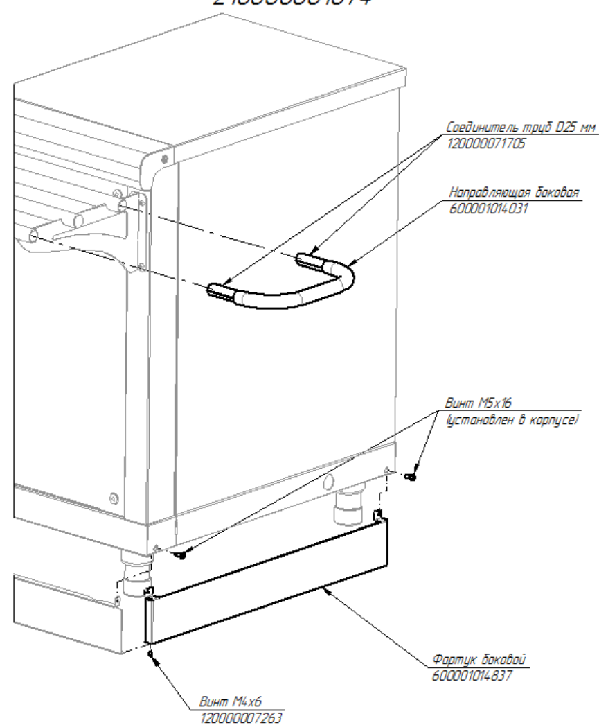
Рис.3 Комплект торцевой
